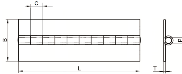
Art. M27/ 0027 Cerniere al metro - Bar Hinges AISI 304
